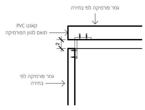
פרט חיבור - זוויתן
