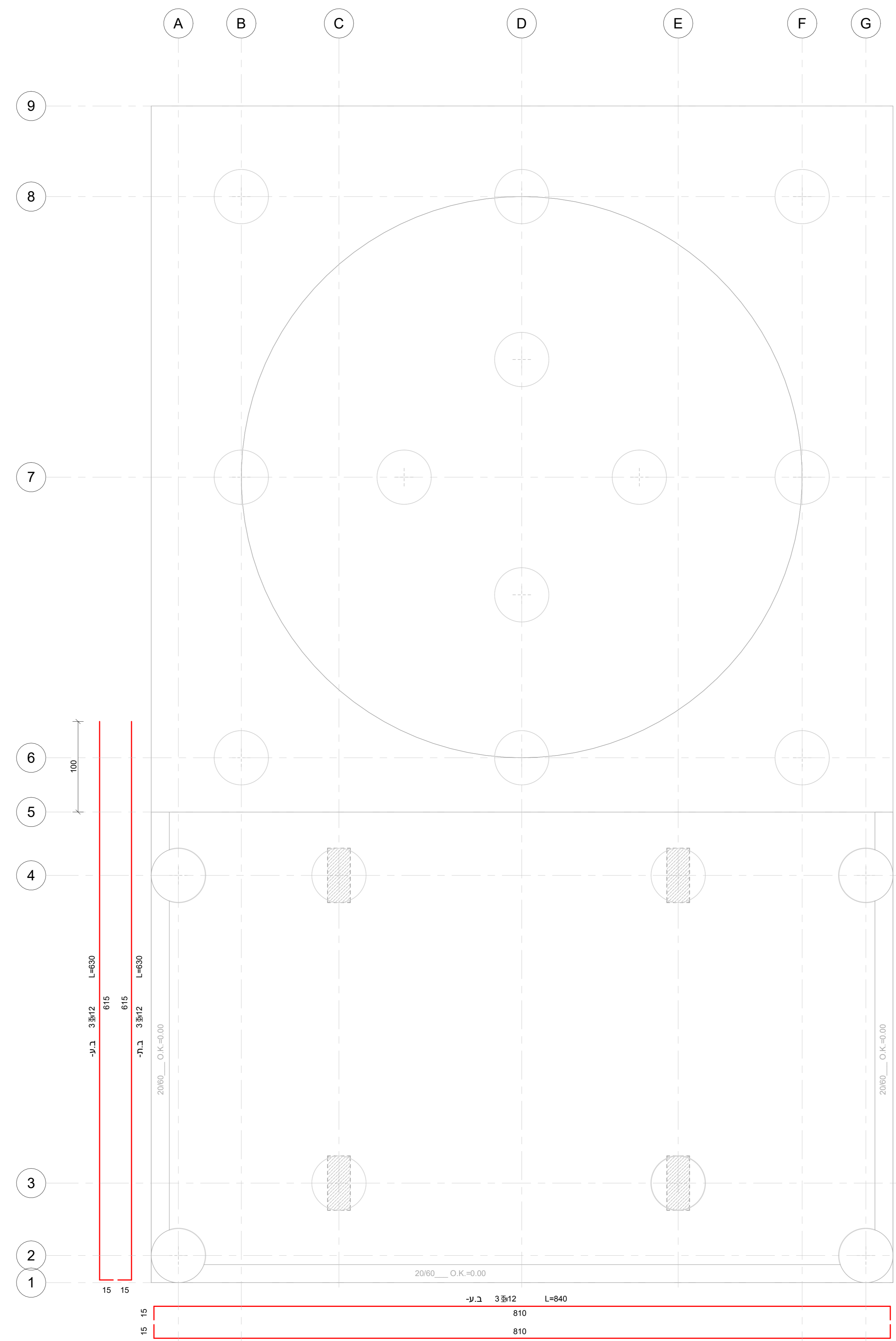
ברזל קורות - ST-110 1:25
