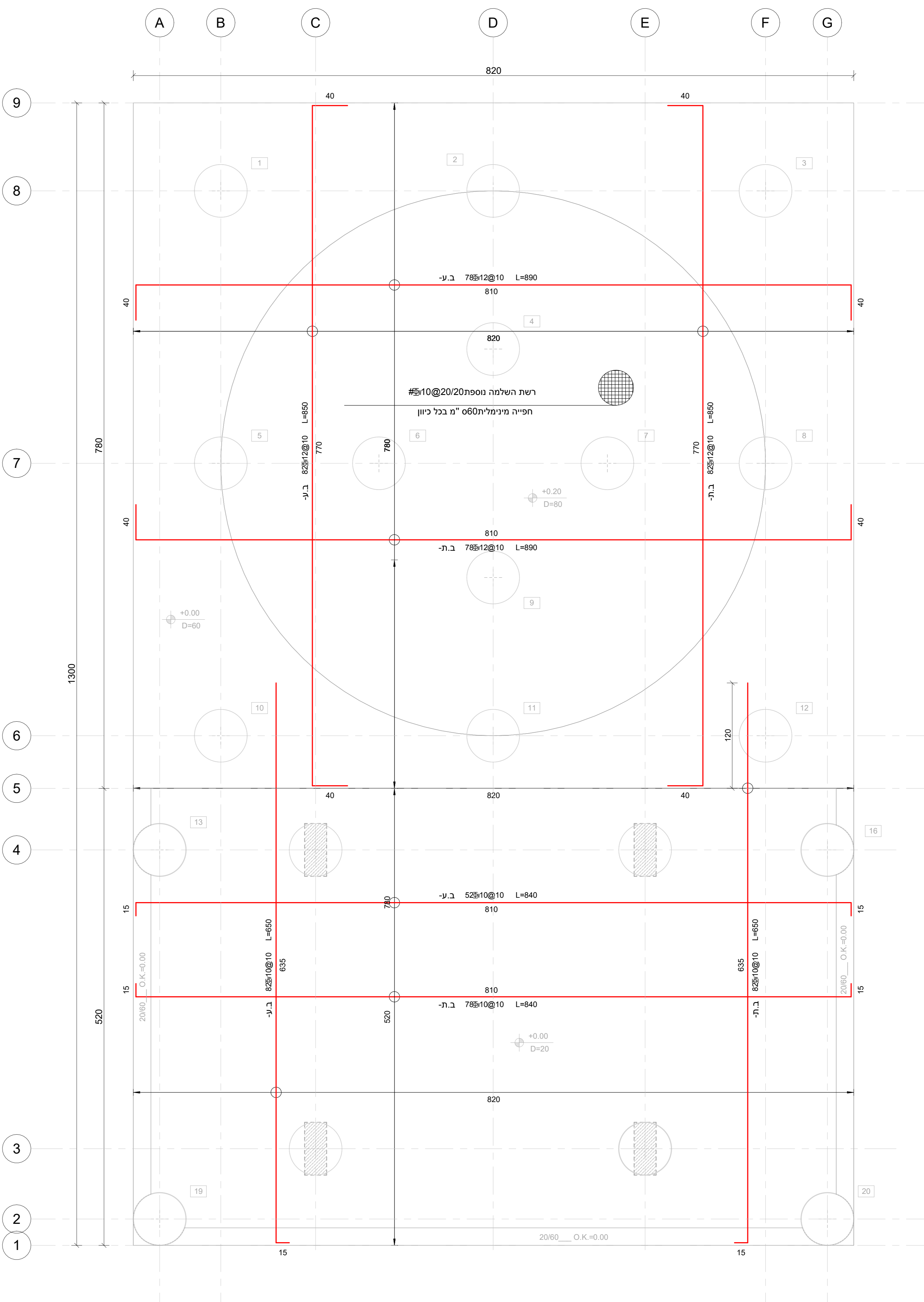
ברזל תחתון ועליון - ST-110 1:25
